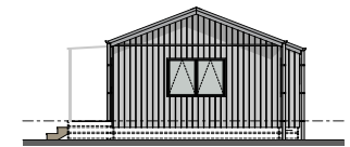
Elevation B
